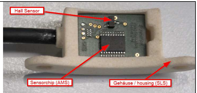
Abb. 3: Sensorchip in Gehäuse mit Hallsensor
