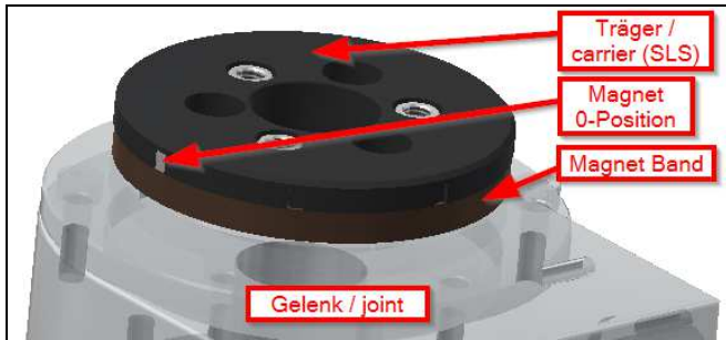
Abb. 2: Magnetring RL-D-20 mit „Südpol“
